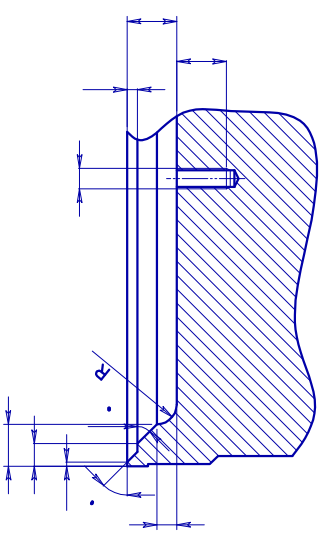
Sez B-B Fuori Scala
