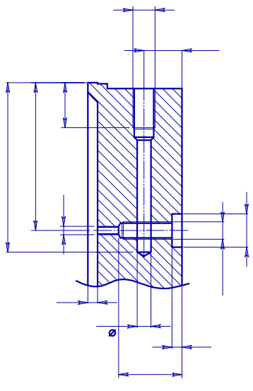
Sez C-C Fuori Scala
